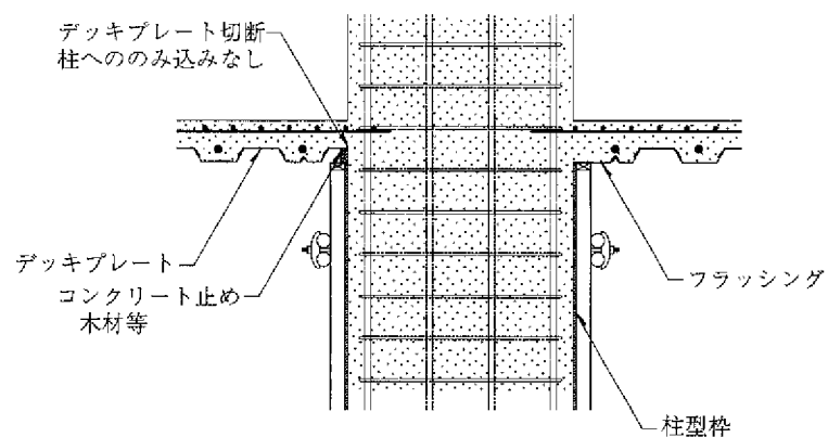
a-a 断面図
