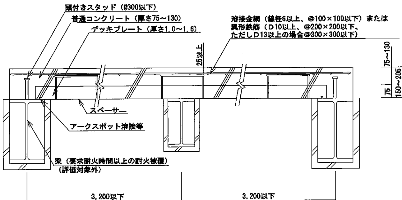
A-A断面図
