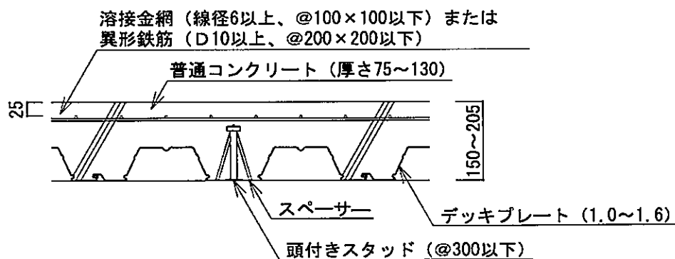
B-B断面図 (デッキプレート中間部梁の場合)
