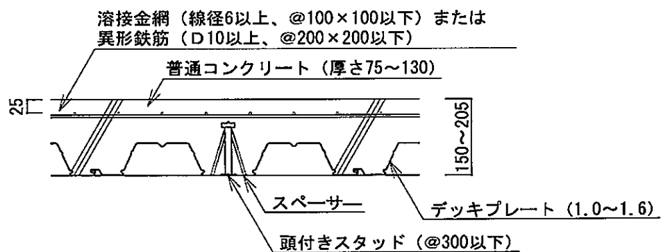
B-B断面図
