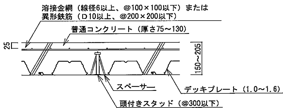
B-B断面図 (デッキプレート端部梁の場合)
