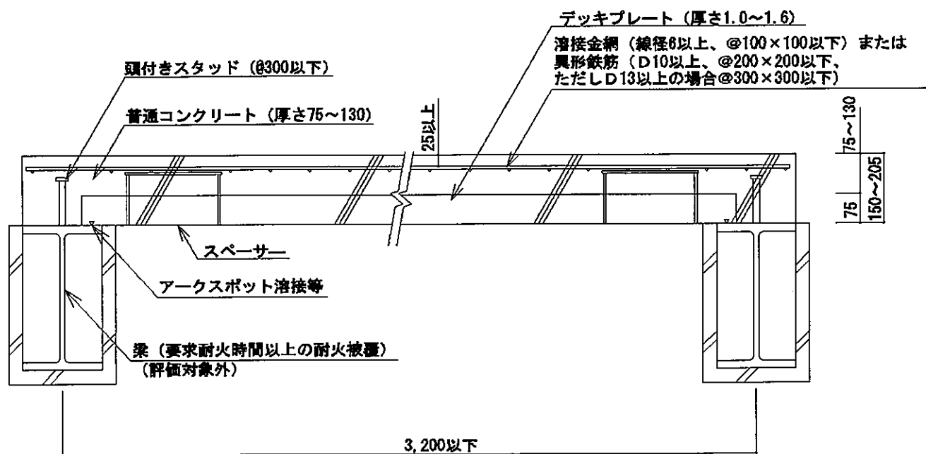
A-A断面図
