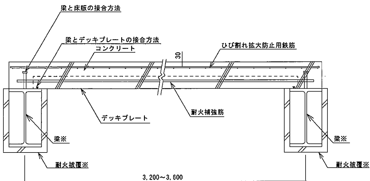
A-A 断面図
