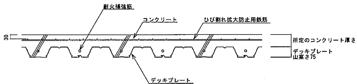
B-B 断面図
