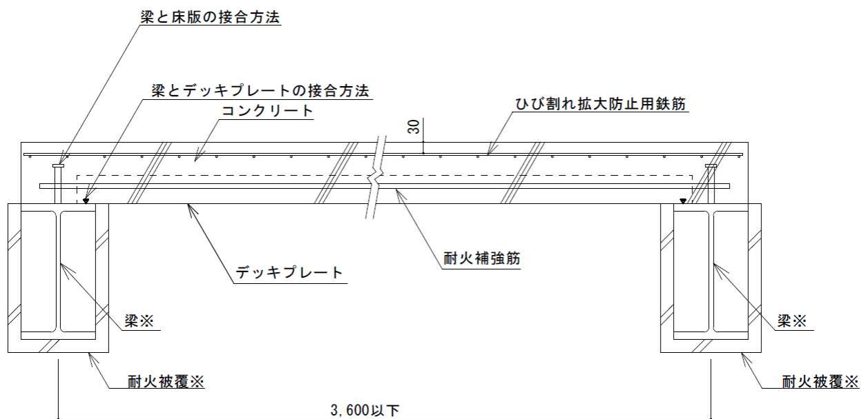
A-A 断面図
