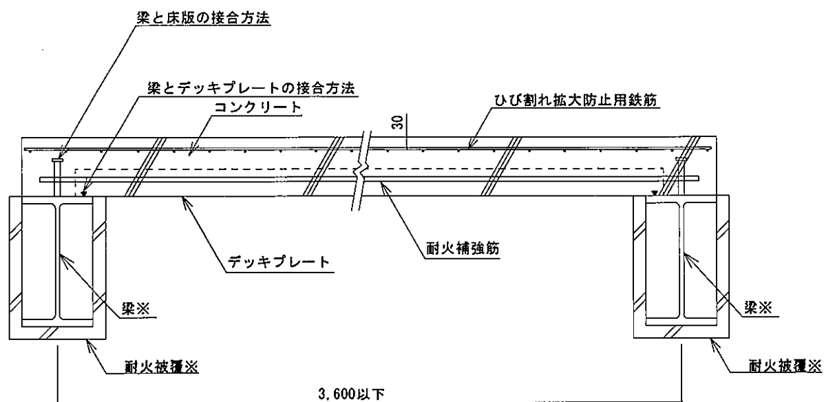
A-A 断面図
