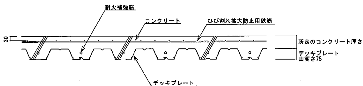
B-B 断面図
