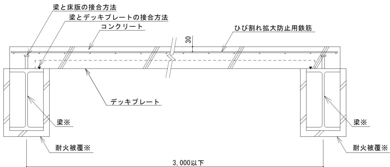
A-A 断面図
