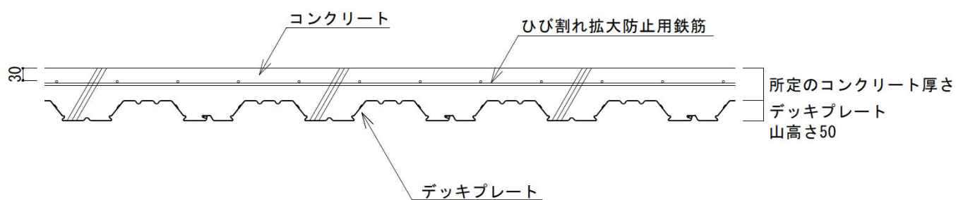
B-B 断面図
