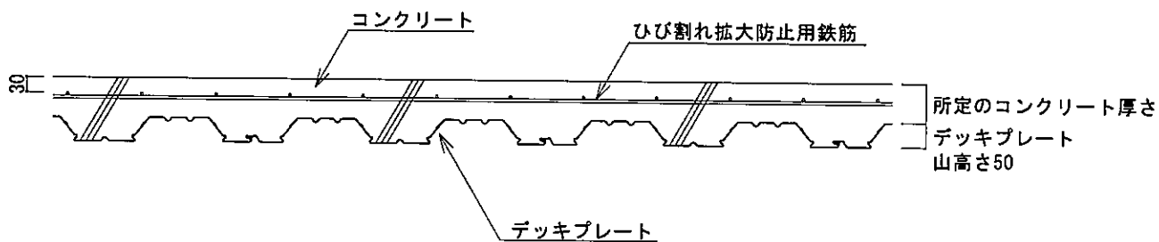
A-A 断面図
