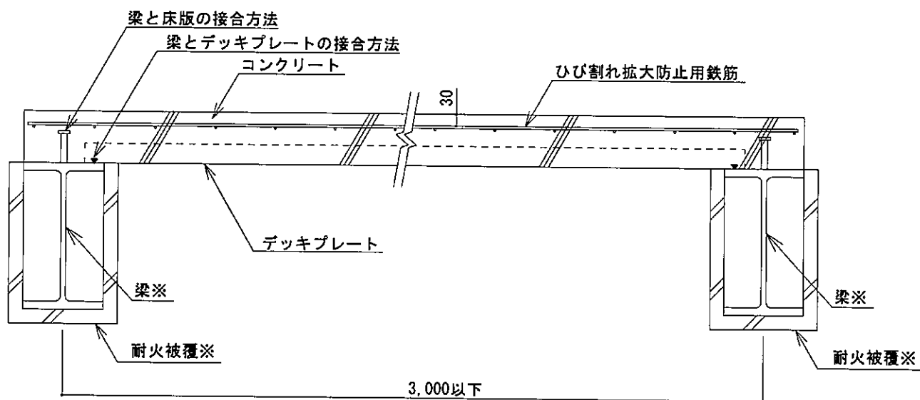
A-A 断面図
