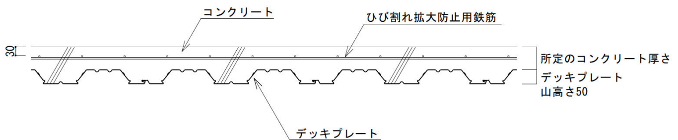
B-B 断面図
