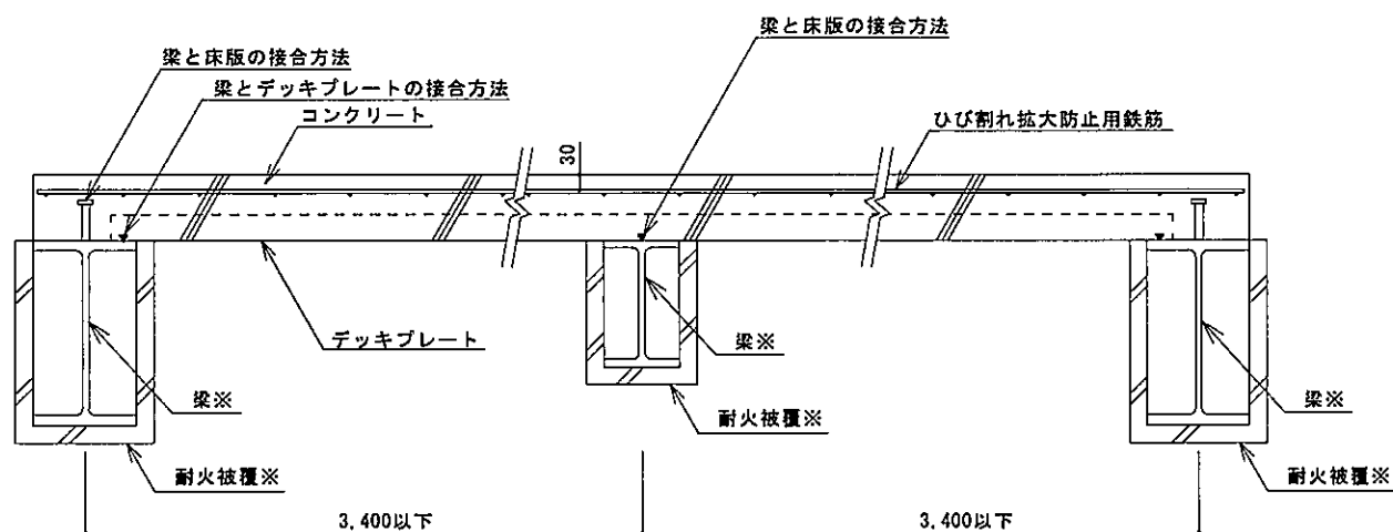
A-A 断面図
