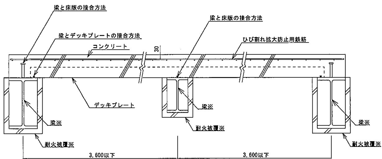
A-A 断面図
