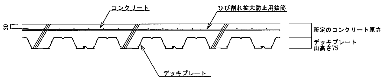
B-B 断面图
