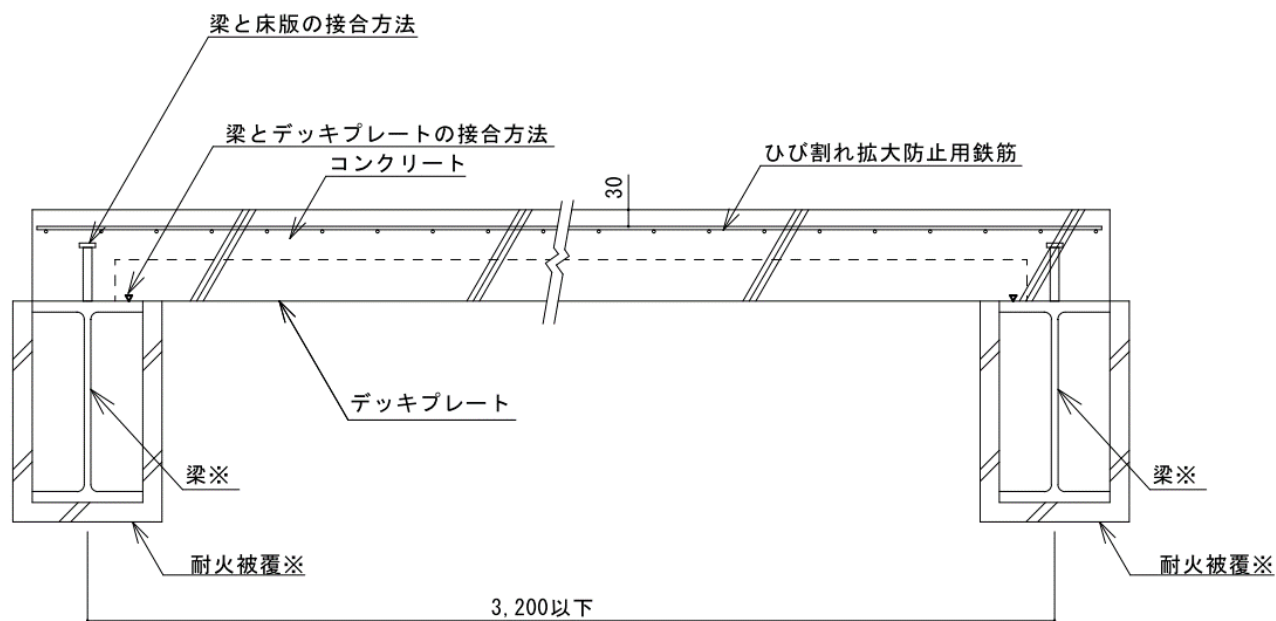
A-A 断面図
