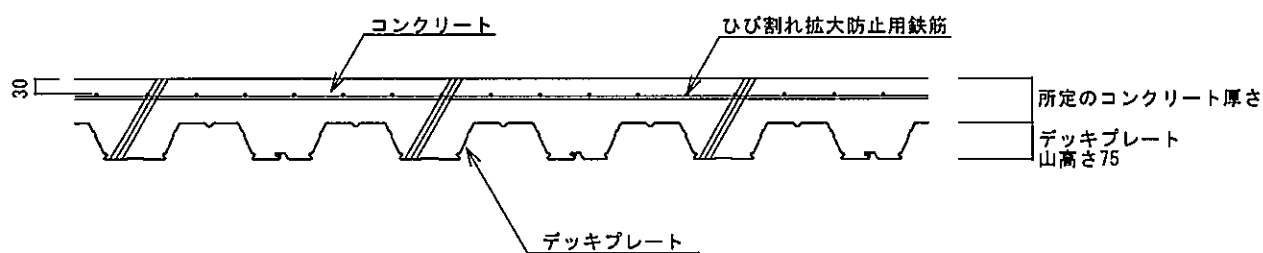
B-B 断面图
