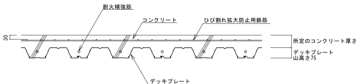
B-B 断面図
