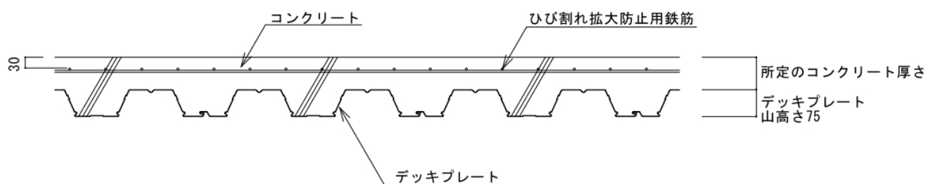
B-B 断面図
