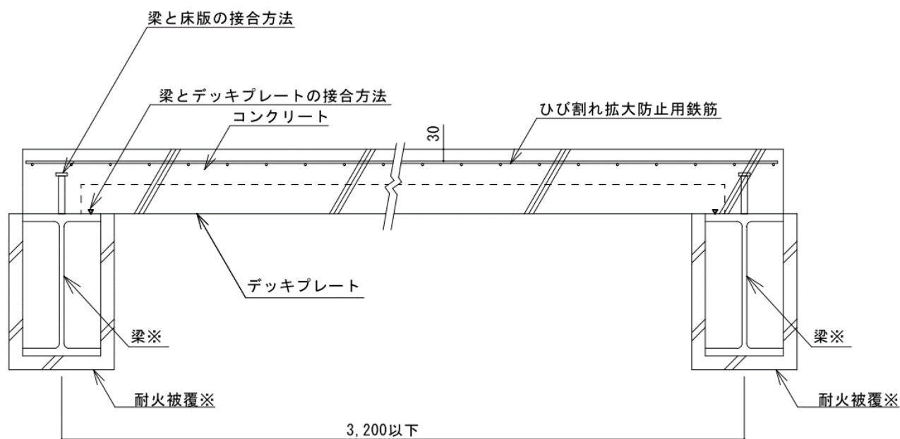
A-A 断面図
