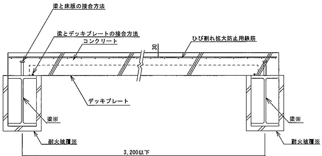
A-A 断面图
