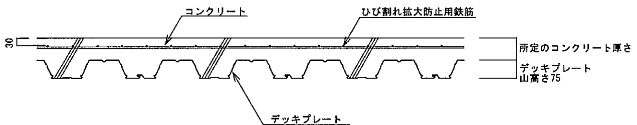
B-B 断面图
