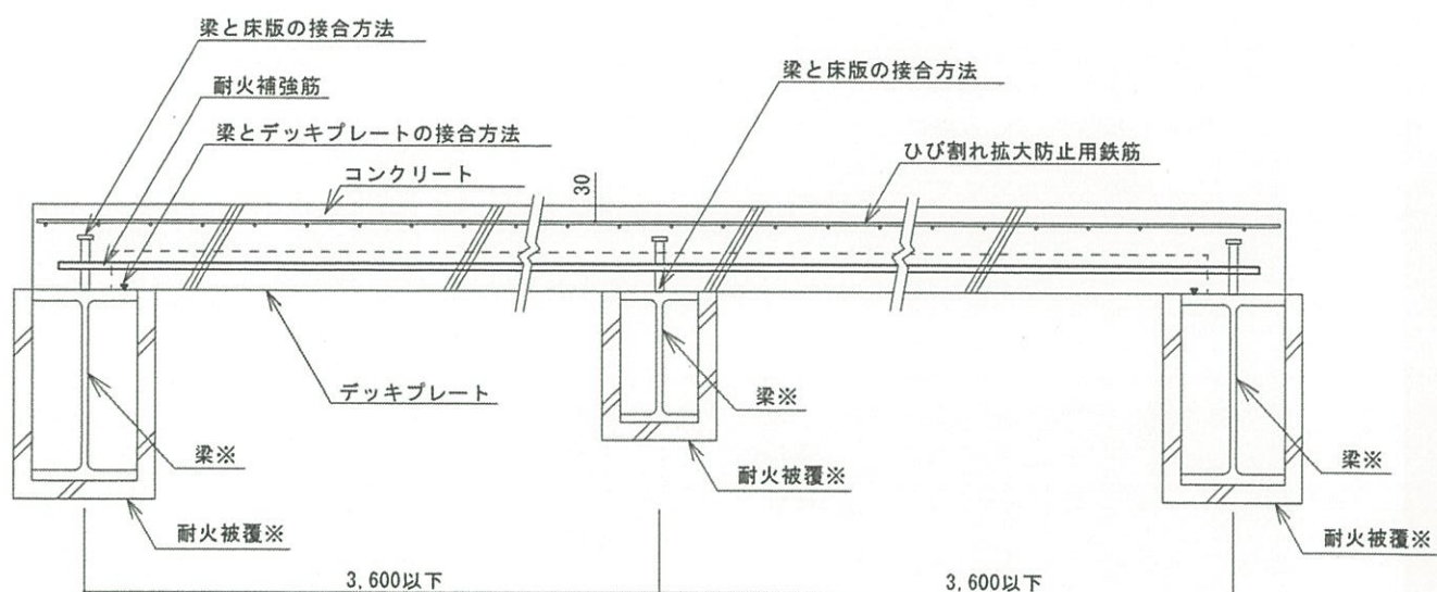
A-A 断面図
