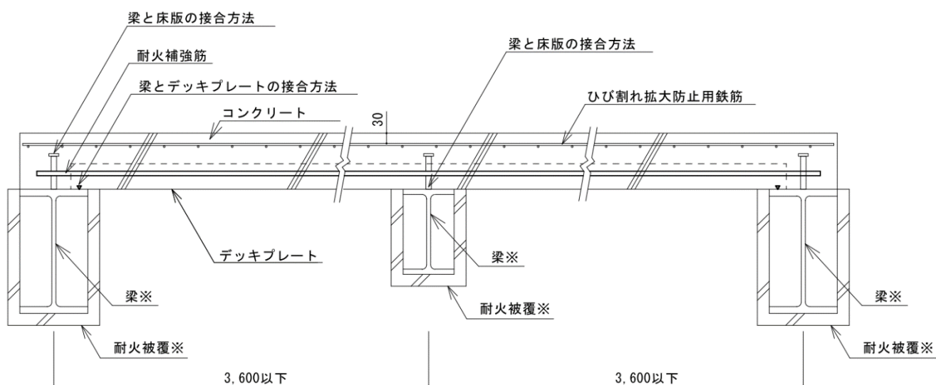
A-A 断面図
