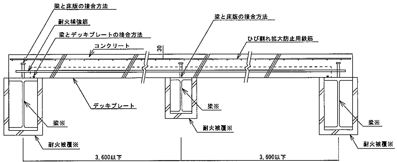
A-A 断面図
