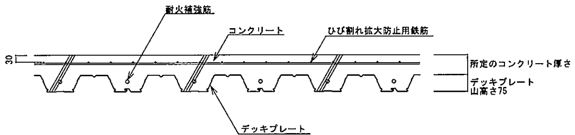
B-B 断面図
