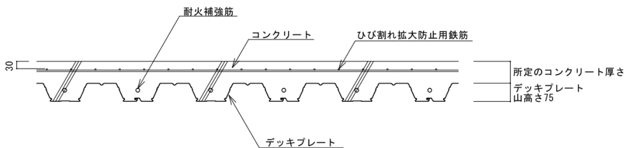
B-B 断面图
